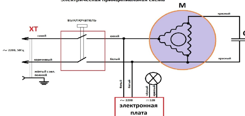
Электрическая принципиальная схема
