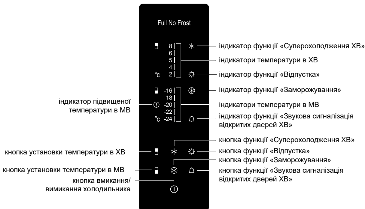
Рисунок 3 — Блок управління
