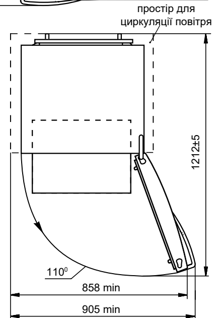
Рисунок 2 — Холодильник (вигляд зверху)
