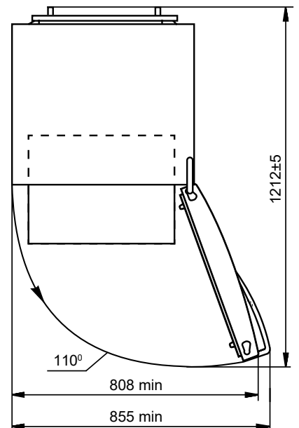
2-сүрөт — Муздаткыч (үстүнөн карагандагы көрүнүш)
