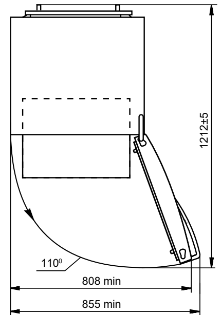
Şəkil 2 – Soyuducu (üstədən görünüşü)
