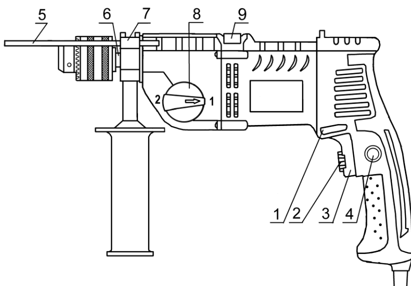
Рис.1 Устройство машины
