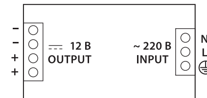
Рис. 1.2 Схема подключения блоков питания:
