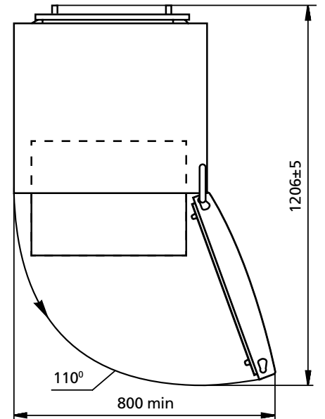
Şəkil 2 — Soyuducu (üstəndən görünüşü)
