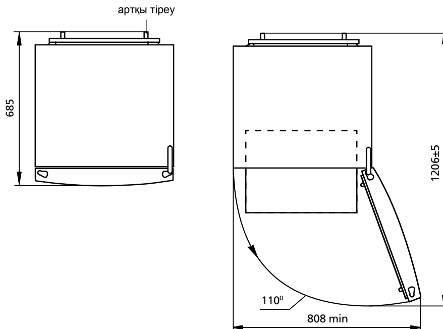
2 сурет — Тоңазытқыш (жоғарыдан көрінетін түр)
