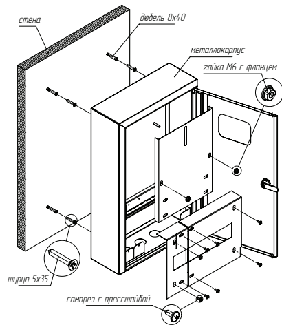
Рис. 1 - Схема монтажа
