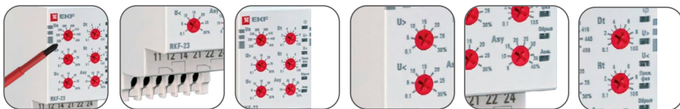
Простая настройка 2 перекидных контакта Отображение неисправности на 5 светодиодах Расширенный диапазон настройки напряжения Возможность настройки асимметрии 2 временных настройки
