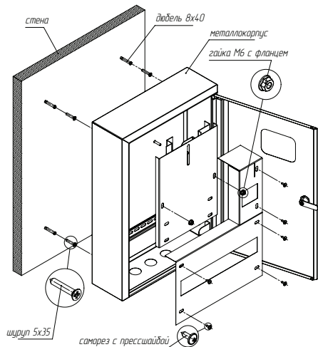
Рис.1. Схема монтажа
