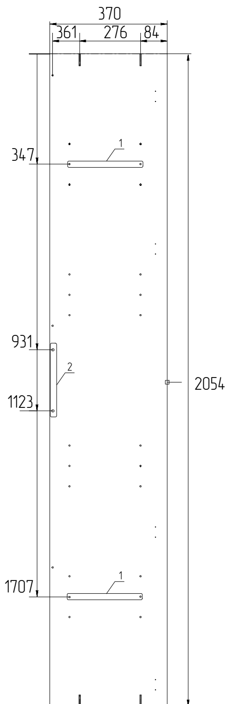
Деталь №2
